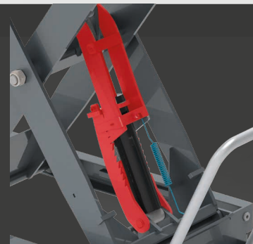
mech. Fallsicherung
